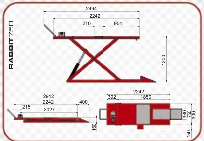
DISEÑOS TÉCNICOS
