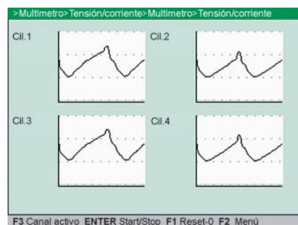
Curva de evolución del vacío para evaluación del control mecánico del motor
